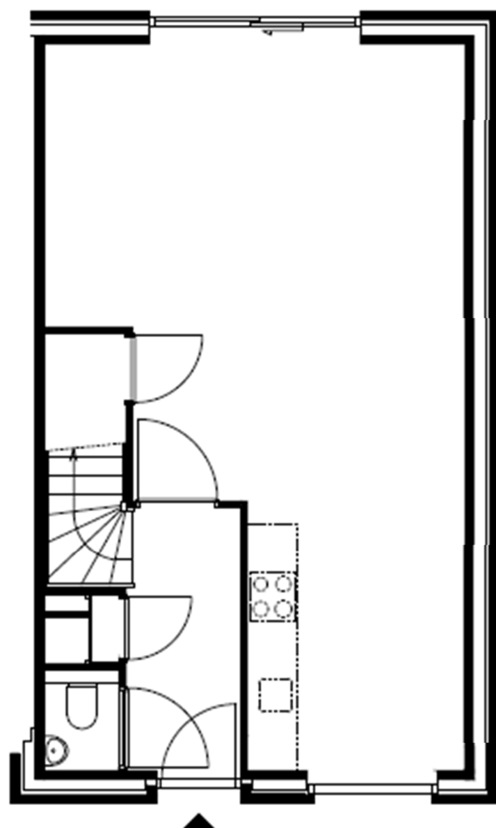
Begane grond
