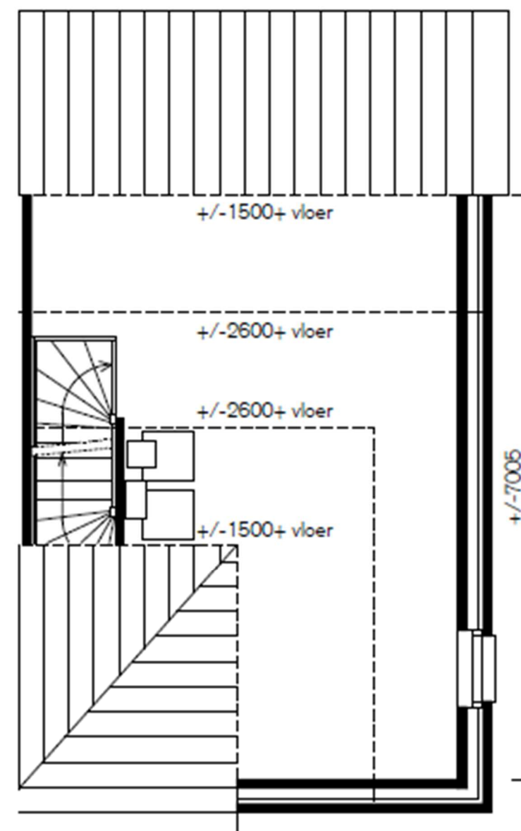
Tweede verdieping
