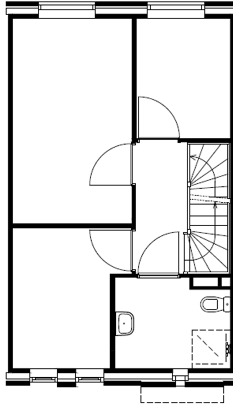
Eerste verdieping
